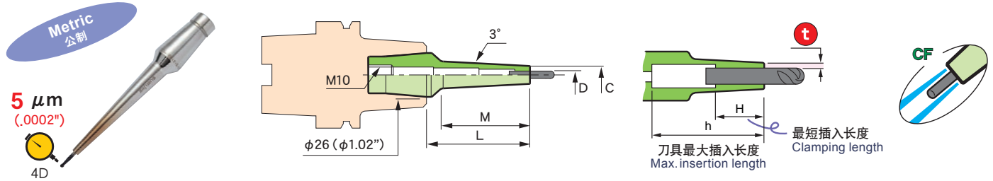
细长型 Slim-type
